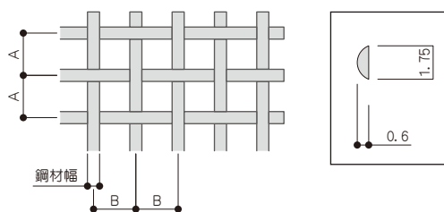
規格寸法表
